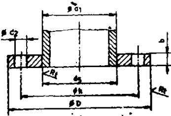
Tip A İşlenmemiş Tip B İşlenmiş (Pürüzlülük R_1=160 )
