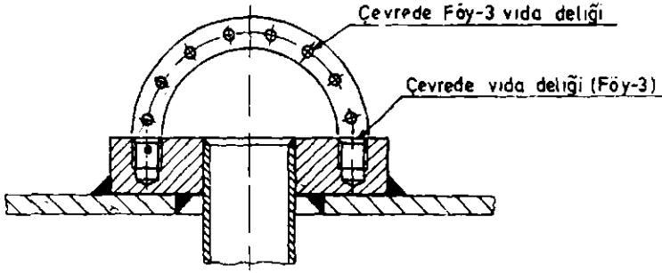
Örnek bağlama şekli
